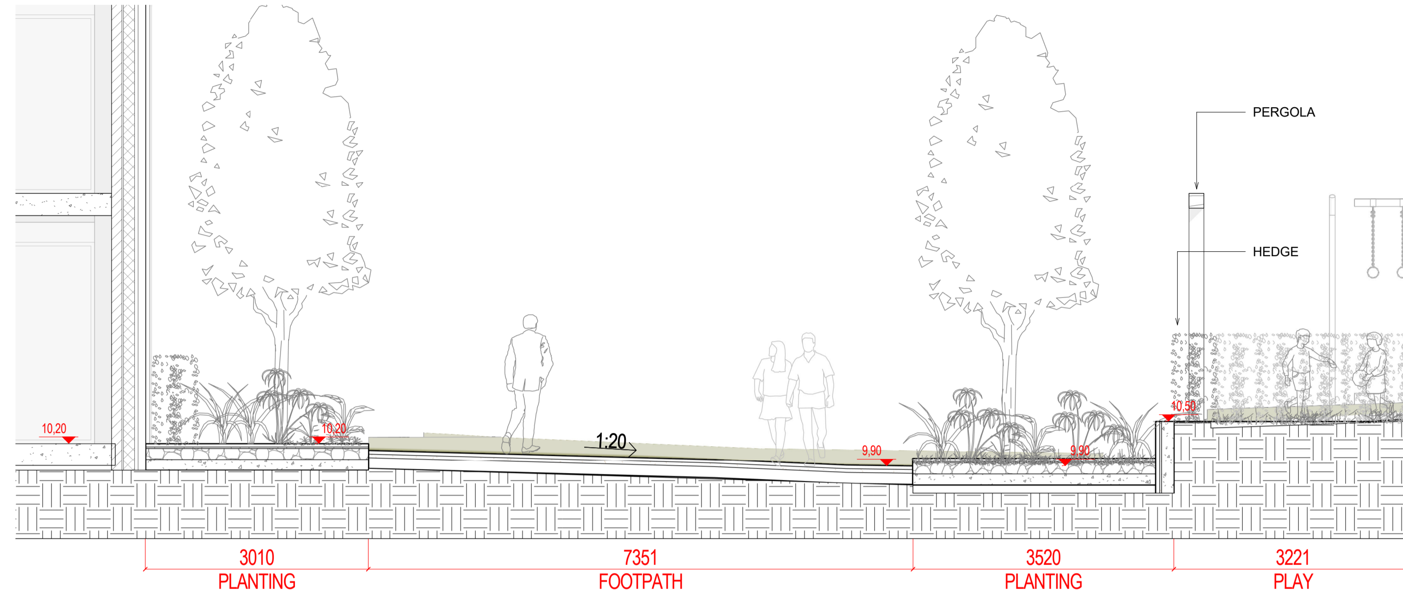
2 SECTION 59 1:50 @A1
