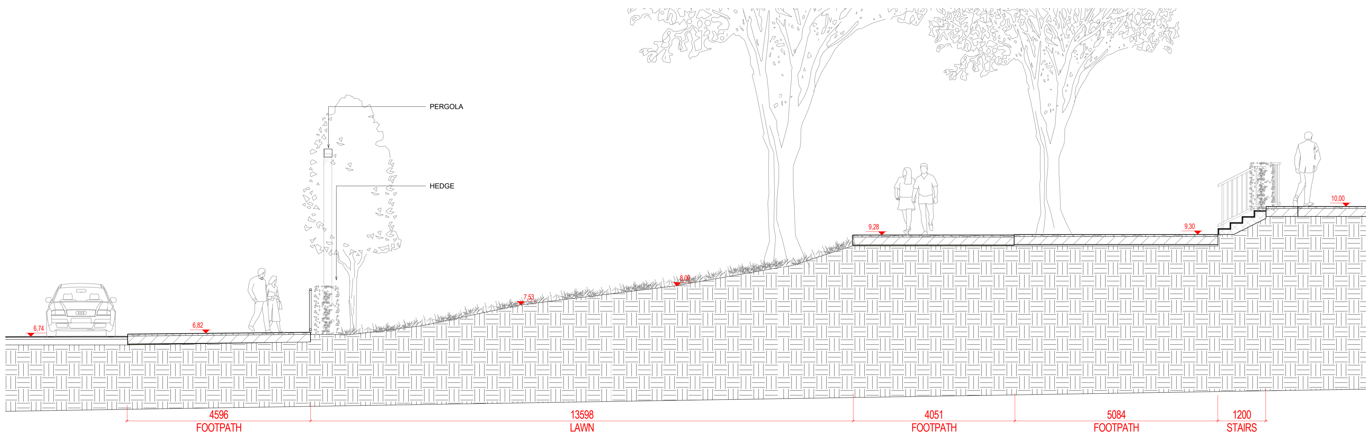
3 SECTION 60 1:50 @A1
