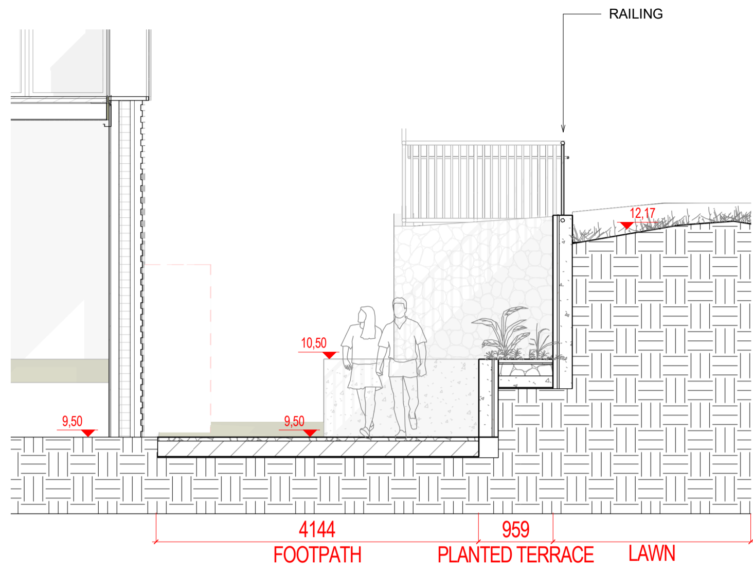
1 SECTION 58 1:50 @A1
